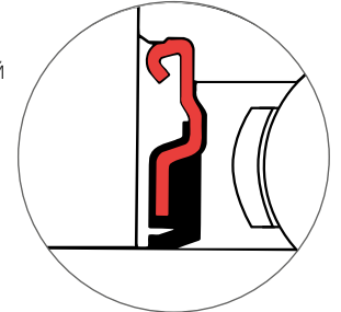
Однокромочное (стандартное) уплотнение
